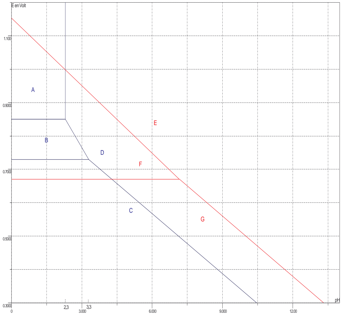
Figure I. Diagrammes E-pH simplifiés du mercure et de l'iode
